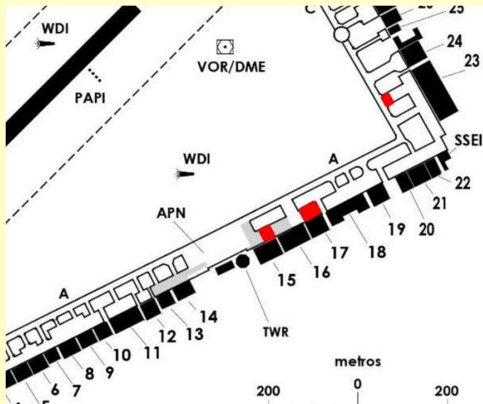
Gráfico 2. Ampliación del plano de Aeródromo San Fernando, sector plataformas con pavimento flexible de hangares 15 y 17 con restricción para todas las operaciones de aeronaves, vehículos y personas.
