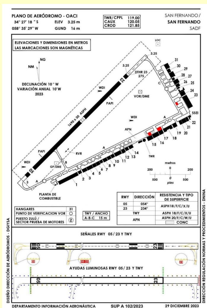
Gráfico 1. Sectores restringidos para todas las operaciones en plataformas de pavimento flexible de hangares 15 y 17, y calle de acceso al hangar 23 clausurada del Aeropuerto Internacional San Fernando.
